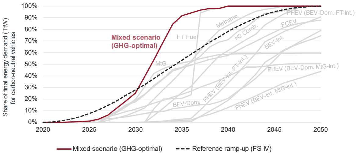
Abbildung 1: Anteil THG-neutraler TtW Energiebedarf im THG-optimal technologieneutralen Mix-Szenario; Einzeltechnologieszennarien in grau hinterlegt.
